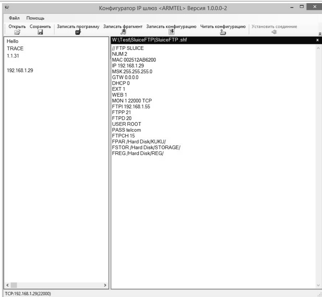
Рисунок 5 – Программа конфигулятора IP-шлюза
