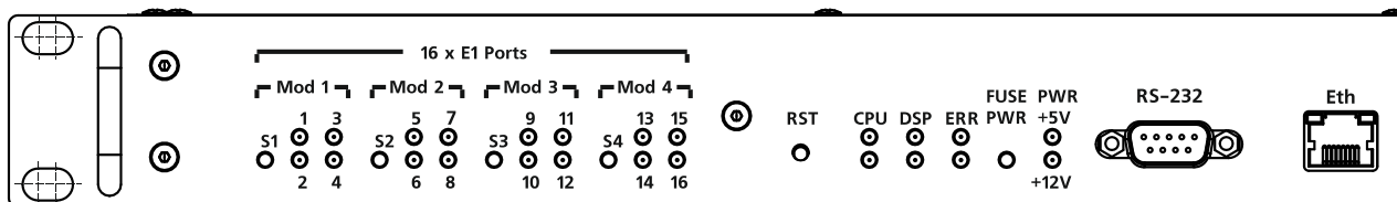
Рисунок 5 – Фрагмент лицевой панели DCN-2
