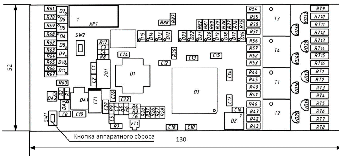
Рисунок 7 – Внешний вид платы 4Е1
