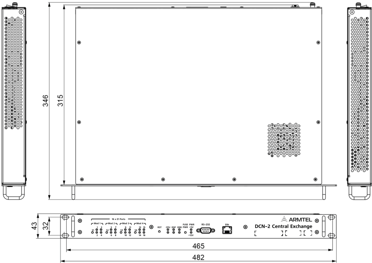
Рисунок 1 – Внешний вид и габаритные размеры DCN-2
