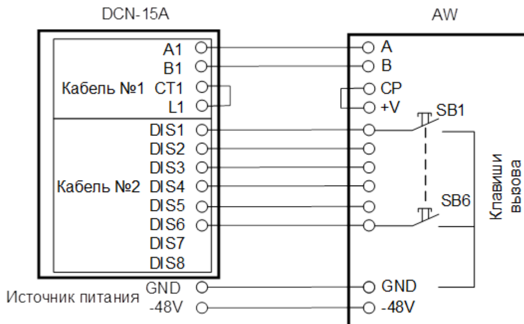
Рисунок А.2 – Подключение к DCN-15A аналогового абонентского переговорного устройства
