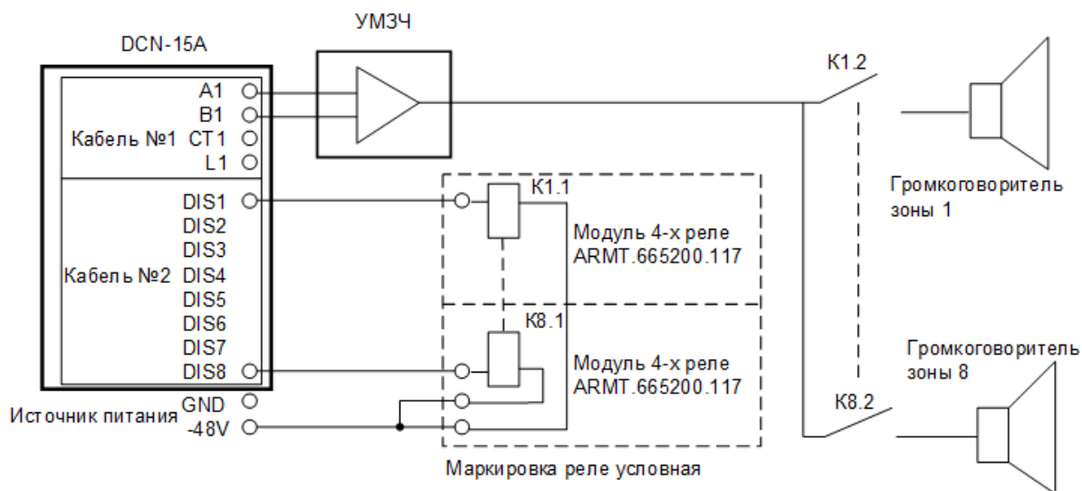
Рисунок А.3 – Построение системы зонального оповещения
