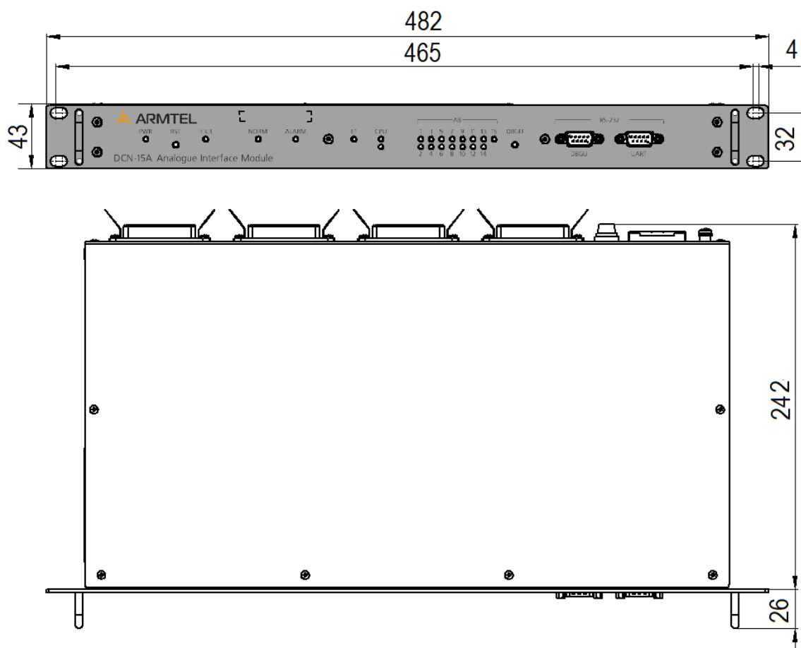
Рисунок 2 – Внешний вид и габаритные размеры DCN-15A
