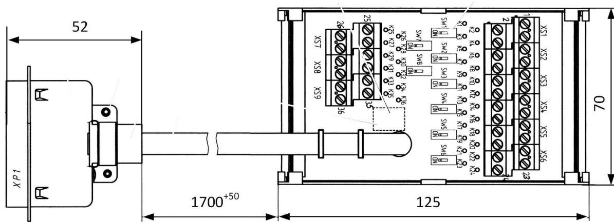
Рисунок А.1 – Кабель подключения DCN-15A
